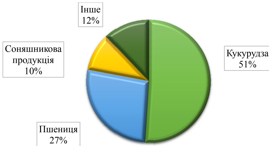
Рис. 1. Експорт зернових культур через Чорноморську зернову ініціативу
