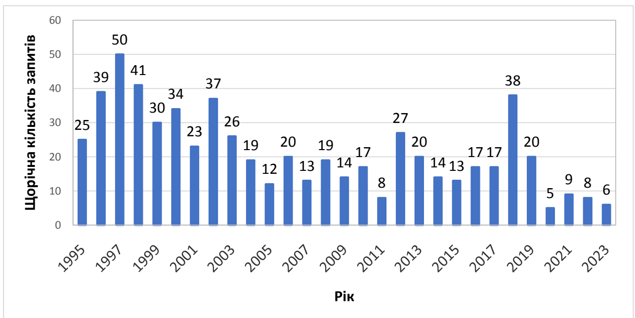
Рис. 1. Динаміка запитів щодо консультацій СОТ у 1995-2023 рр.
